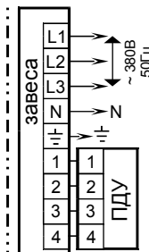
Схема подключения T206E, T209E, T212E, T218E, T309E, T318E к трёхфазной сети и ПДУ.
