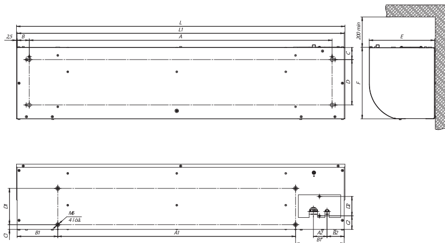
РИС. 4 Установочные размеры ZVV-1E6T, ZVV-1.5E9T, ZVV-2E12T, ZVV-2E18T, ZVV-2E24T
