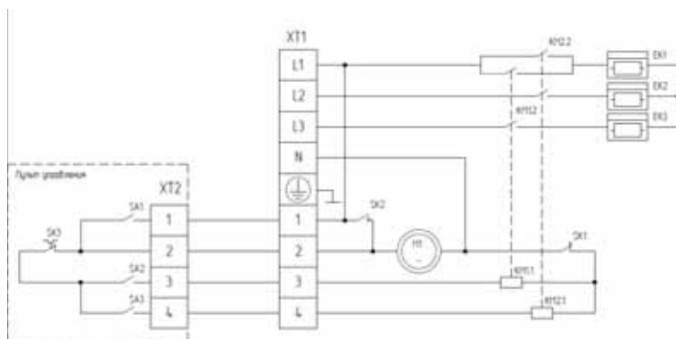
РИС. 6 Схема электрическая ZVV-2E18T, ZVV-2E24T
