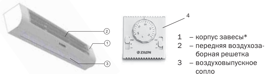
РИС. 1. Тепловая завеса*
