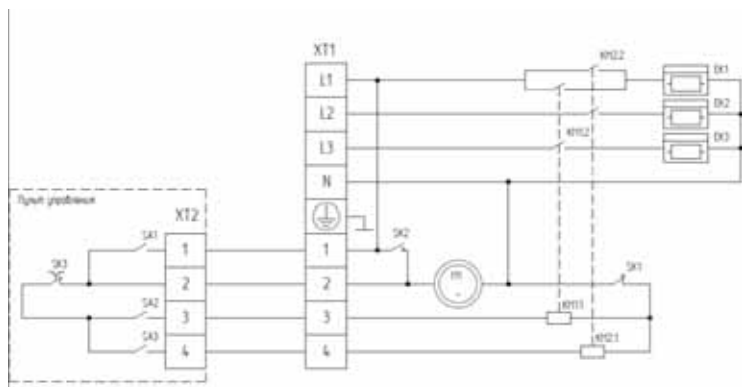
РИС. 5 Схема электрическая ZVV-1E6T, ZVV-1.5E9T, ZVV-2E12T
