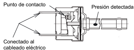
Estructura del preostato de alta presión
